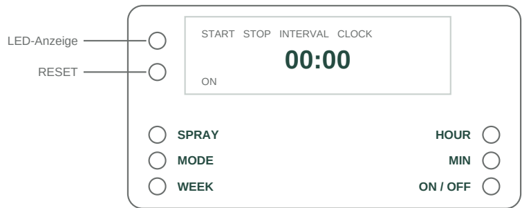
Bedienfeld, schematisch
